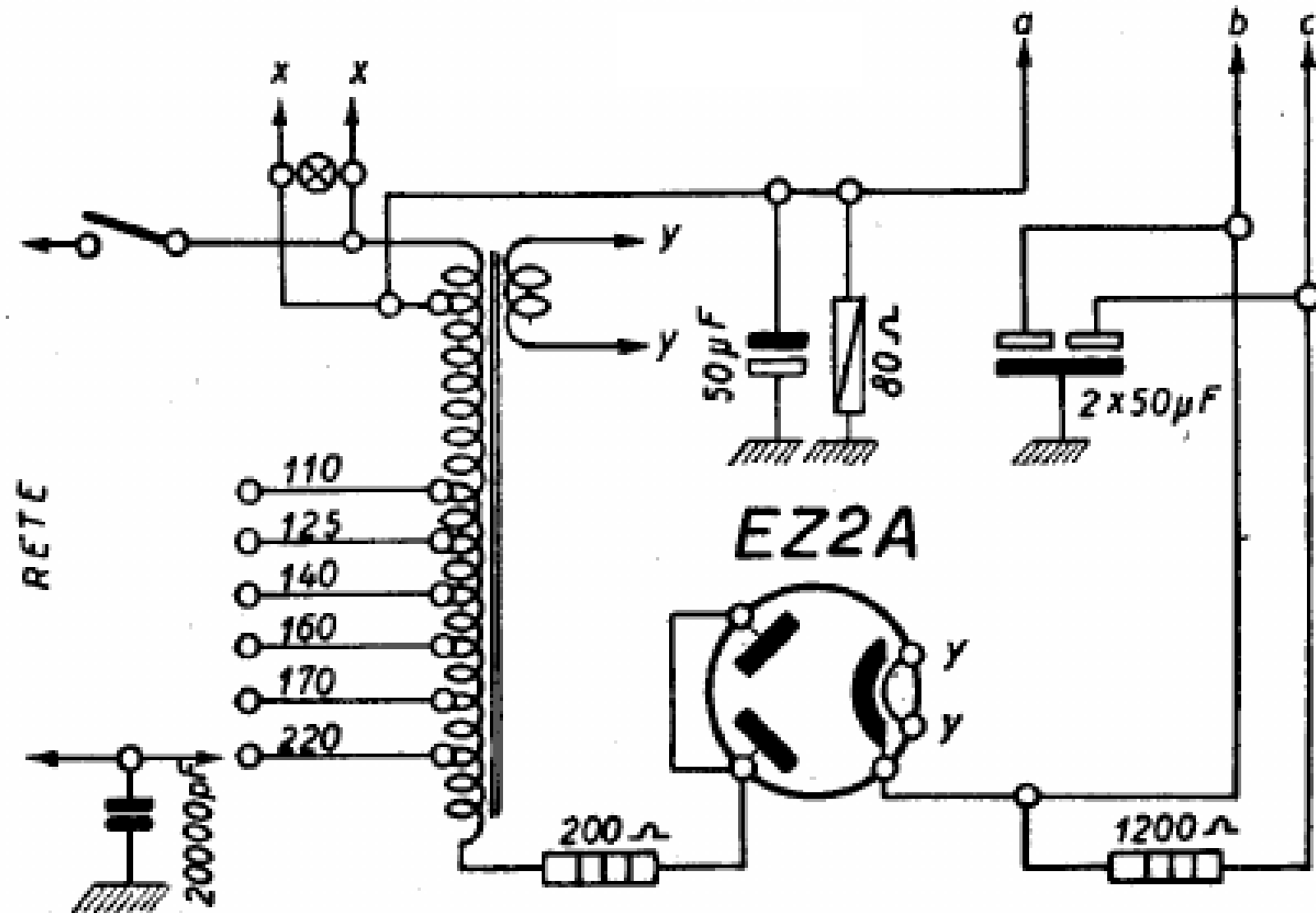
PHILIPS RADIO - Mod. BI 390/A - Variante con elettrolitico da 2 \times 50 \mu\text{F} .
